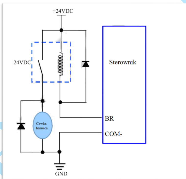
Rys.6. Wyjście hamulca
